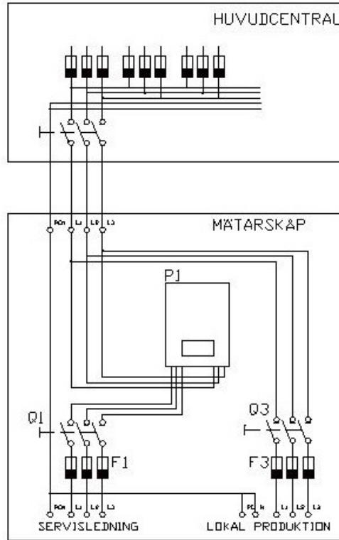
Äldre mätarskåp
