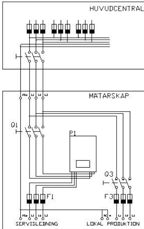
Nytt mätarskåp
